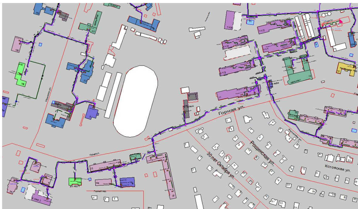
Рисунок Ошибка! Текст указанного стиля в документе отсутствует..39 Результат гидравлического расчета - расчетный путь теплоносителя от котельной Горная, 13 до ПТ-Горная,2а
