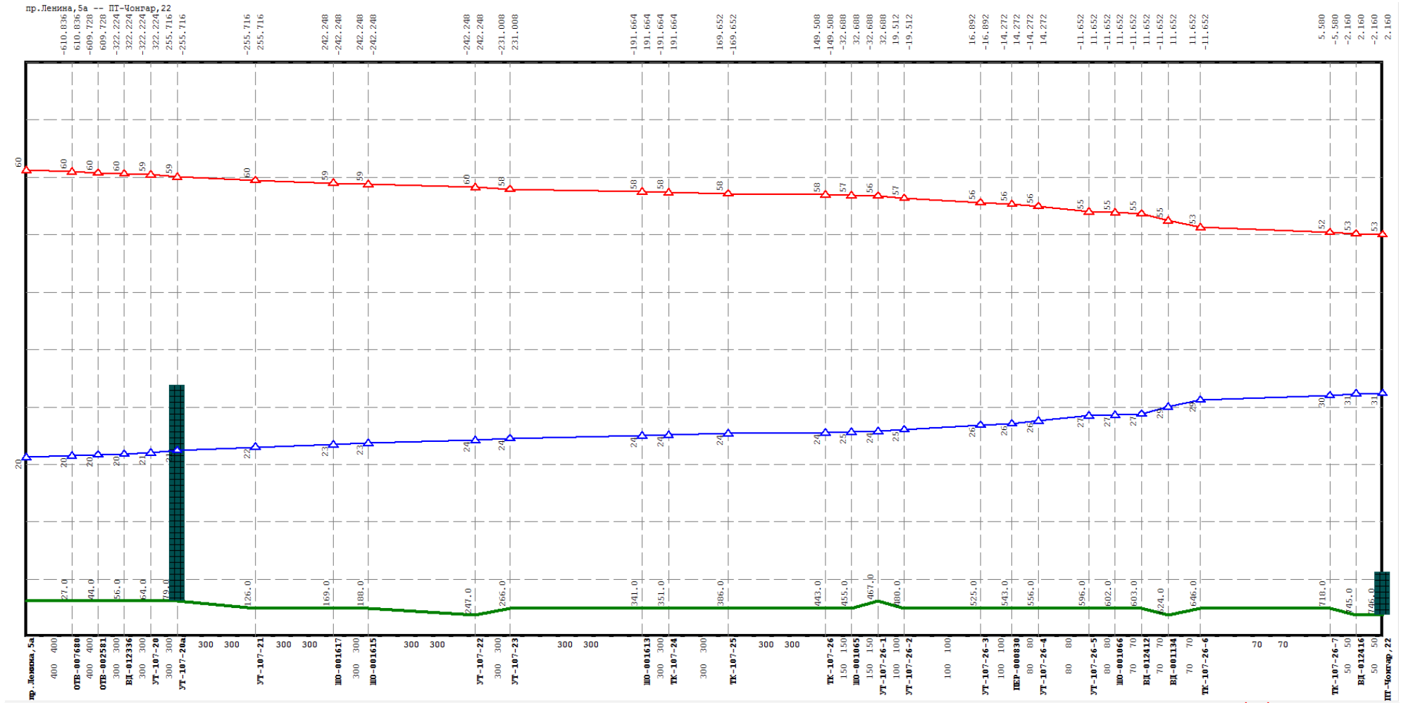
Рисунок Ошибка! Текст указанного стиля в документе отсутствует..18 Результат гидравлического расчета - график гидравлических режимов по пути теплоносителя от котельной пр. Ленина, 5-а до ПТ-Чонгар, 22
