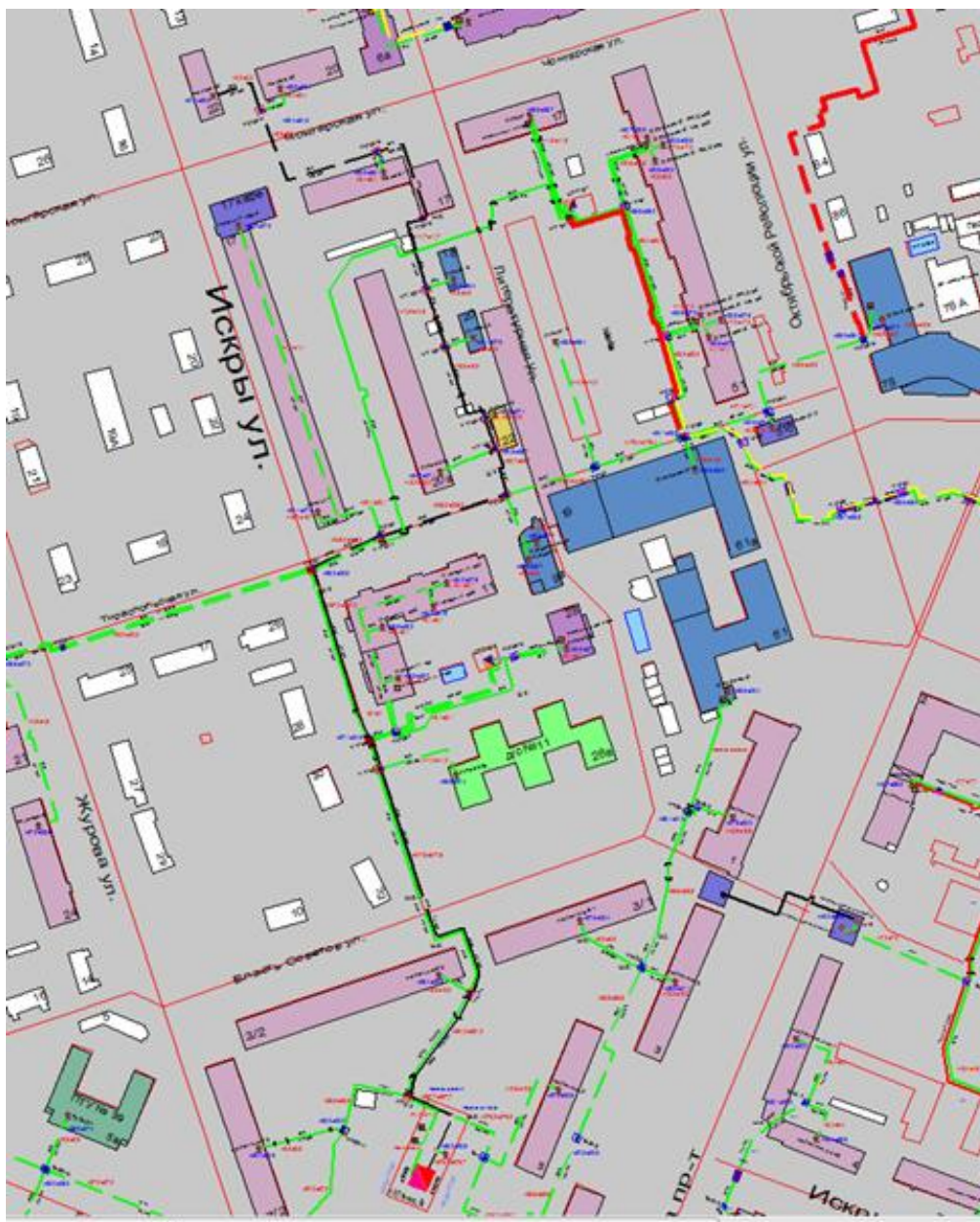
Рисунок Ошибка! Текст указанного стиля в документе отсутствует..17 Результат гидравлического расчета - расчетный путь теплоносителя от котельной пр. Ленина, 5-а до ПТ-Чонгар,22
