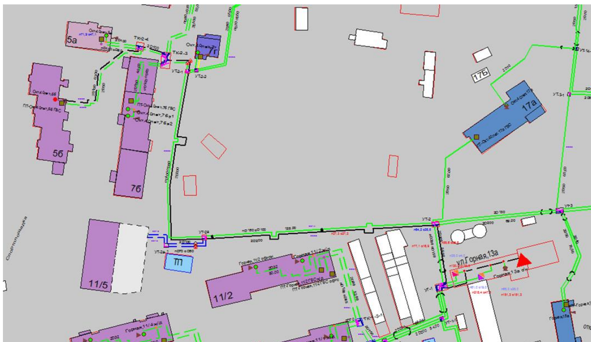
Рисунок Ошибка! Текст указанного стиля в документе отсутствует..41 Результат гидравлического расчета - расчетный путь теплоносителя от котельной Горная, 13 до ПТ-Окт.40лет,5б
