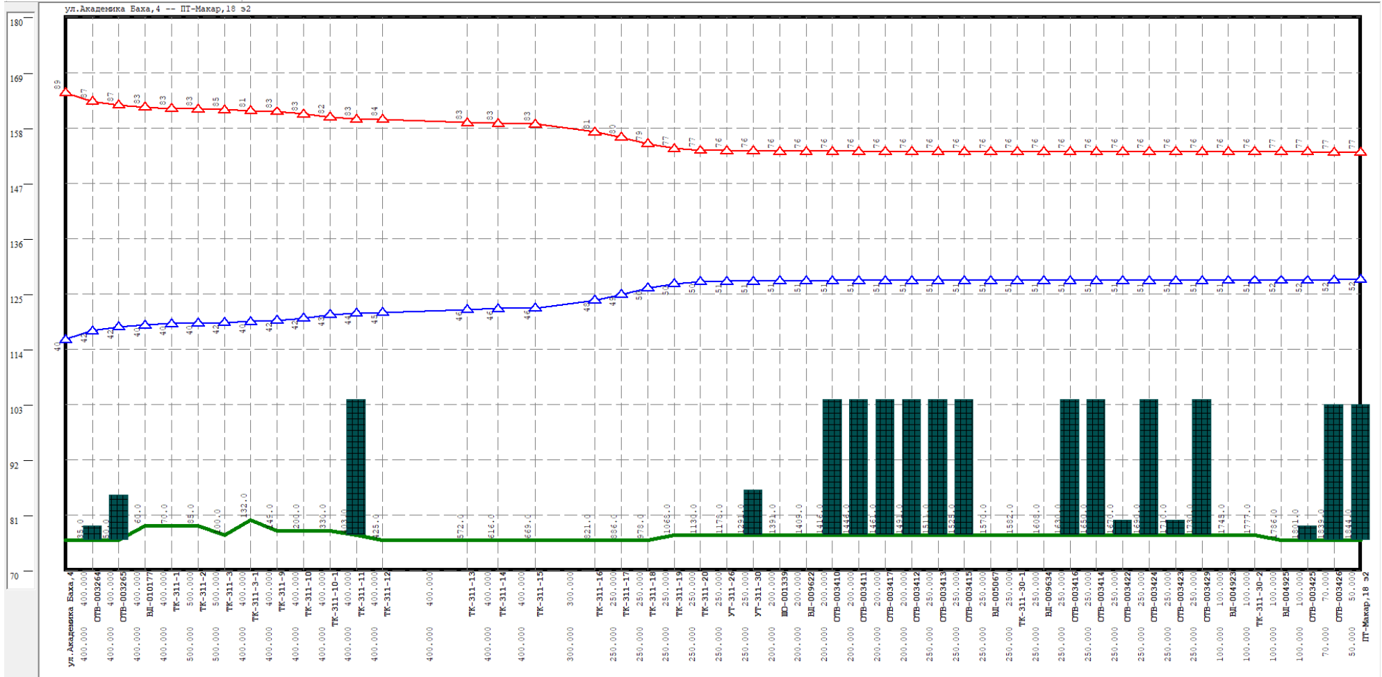
Рисунок Ошибка! Текст указанного стиля в документе отсутствует..10 Результат гидравлического расчета - график гидравлических режимов по пути теплоносителя от котельной Академика Баха, 4-а до ПТ-Макар,18 э2
