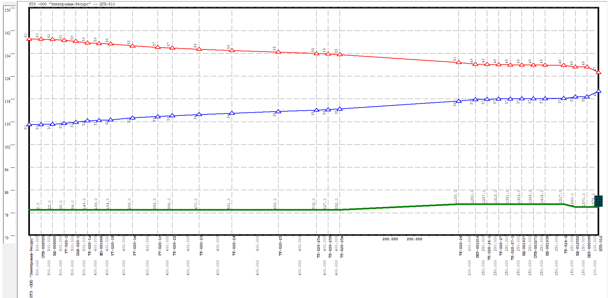
Рисунок Ошибка! Текст указанного стиля в документе отсутствует..94 Результат гидравлического расчета - график гидравлических режимов по пути теплоносителя от котельной Федосеенко, 64 до ЦТП-ул.Федосеен,89а
