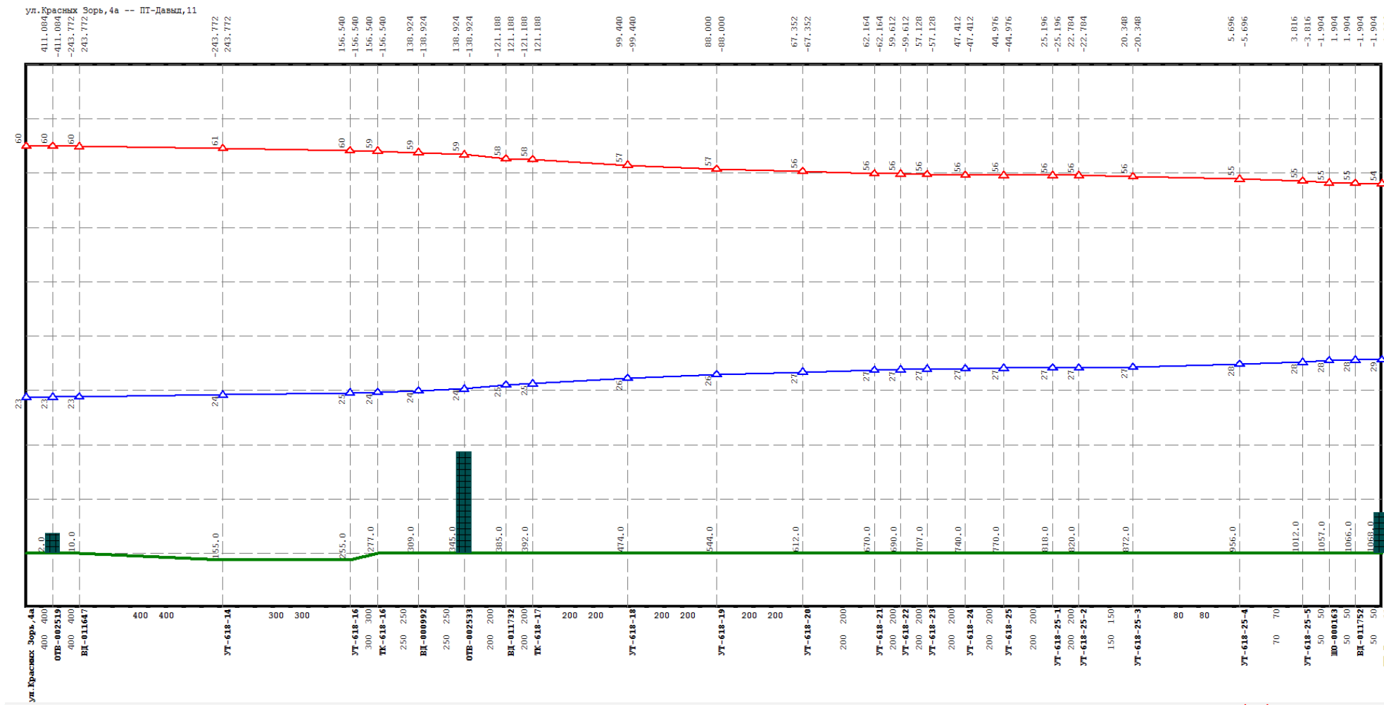
Рисунок Ошибка! Текст указанного стиля в документе отсутствует..78 Результат гидравлического расчета - график гидравлических режимов по пути теплоносителя от котельной Красных Зорь, 4а до ПТ-Давид,11
