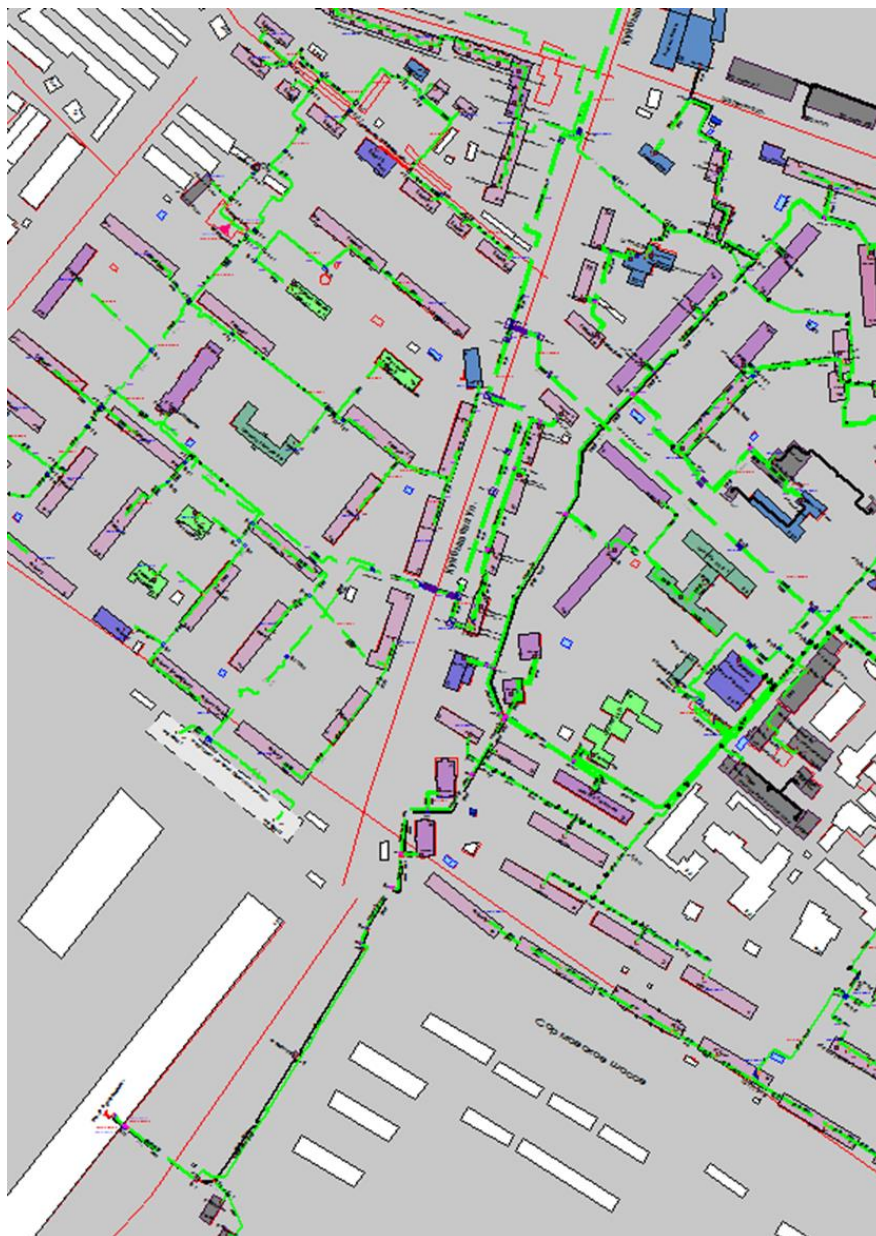
Рисунок Ошибка! Текст указанного стиля в документе отсутствует..115 Результат гидравлического расчета - расчетный путь теплоносителя от котельной Бурнаковский пр., 15 до ПТ-Куйбыш,32,30
