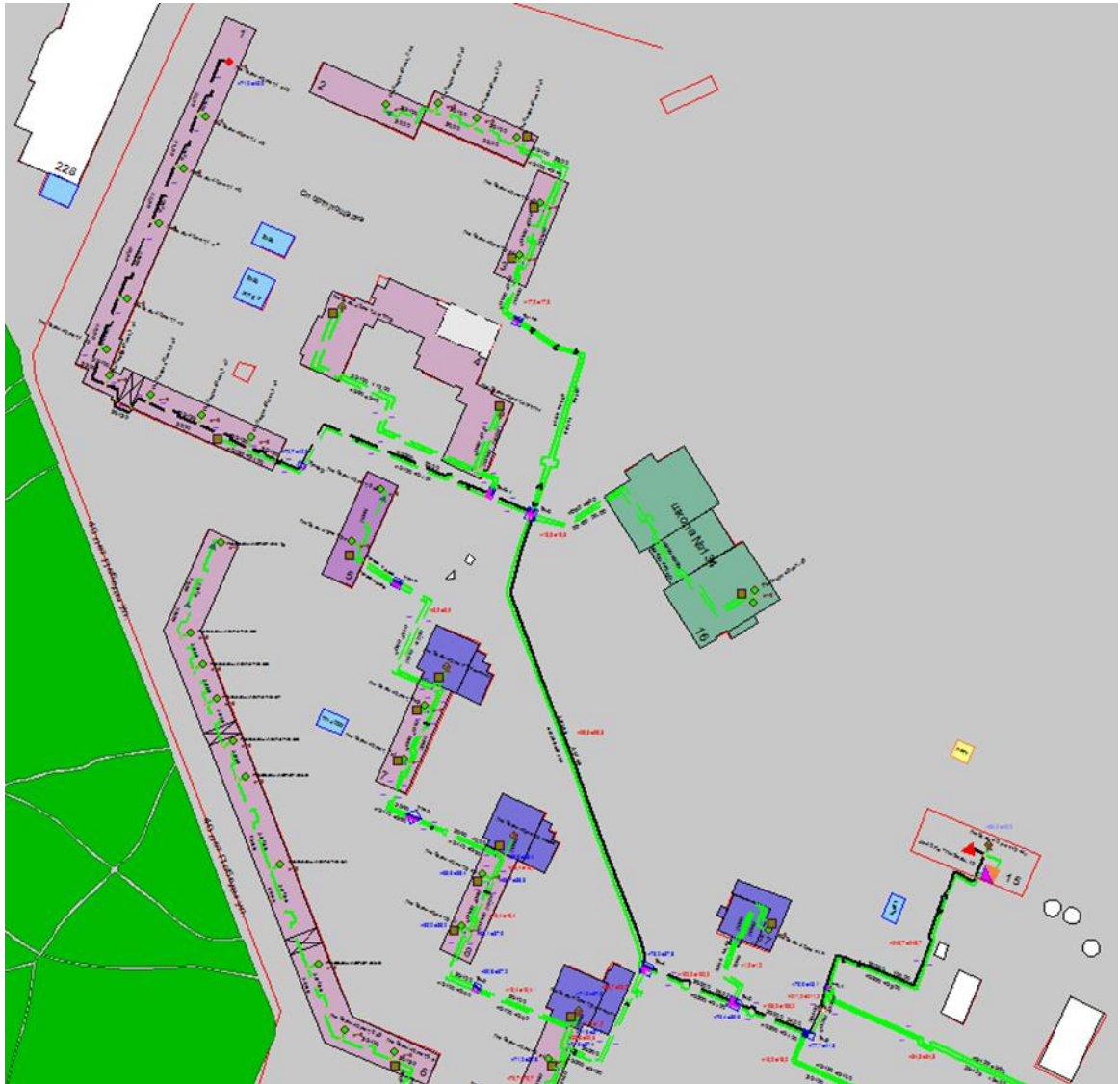
Рисунок Ошибка! Текст указанного стиля в документе отсутствует..43 Результат гидравлического расчета - расчетный путь теплоносителя от котельной 40 лет Победы, 15 до ПТ-Победы 40лет,1 э10
