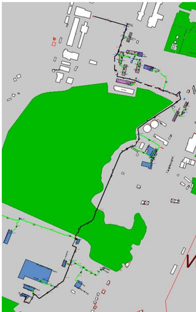
Рисунок Ошибка! Текст указанного стиля в документе отсутствует..97 Результат гидравлического расчета - расчетный путь теплоносителя от котельной Тропинина, 47 до ПТ-Гагар,121 хлор.хоз
