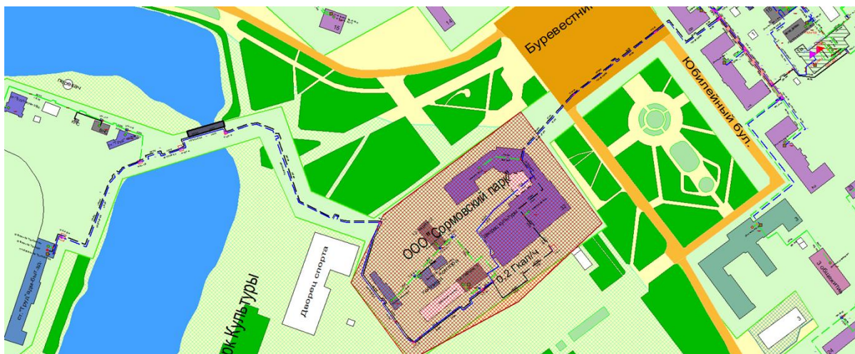
Рисунок Ошибка! Текст указанного стиля в документе отсутствует..3 Результат гидравлического расчета - расчетный путь теплоносителя от котельной Энгельса, 1-в до ПТ-Юбилейн.б-р "Труд"АБК
