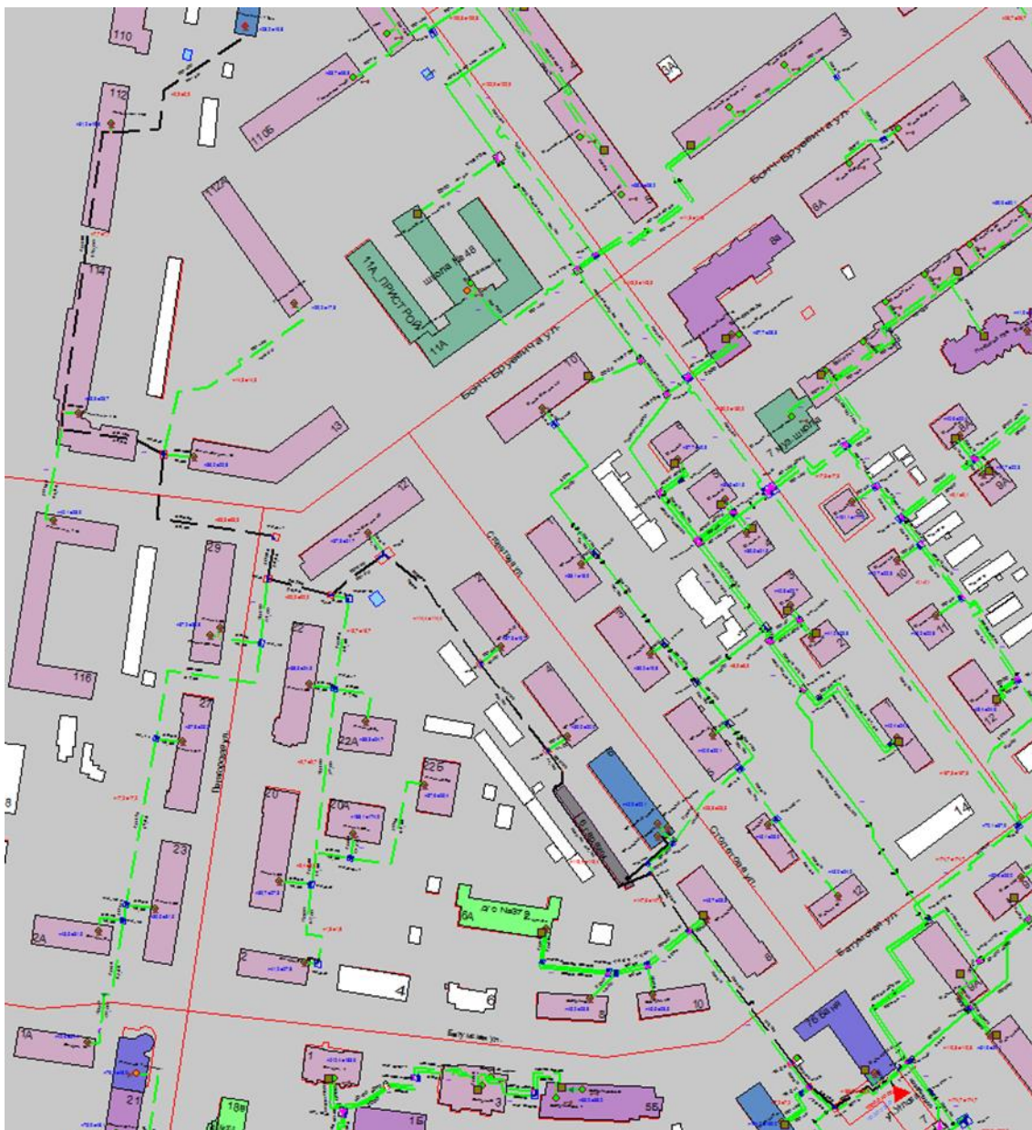
Рисунок Ошибка! Текст указанного стиля в документе отсутствует..105 Результат гидравлического расчета - расчетный путь теплоносителя от котельной Углова, 7 до ПТ-Гагар.пр,110в
