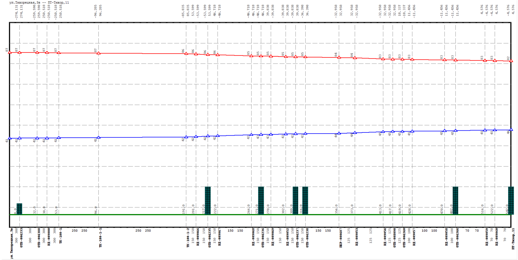
Рисунок Ошибка! Текст указанного стиля в документе отсутствует..84 Результат гидравлического расчета - график гидравлических режимов по пути теплоносителя от котельной Тихорецкая, 3в до ПТ-Тихор,11
