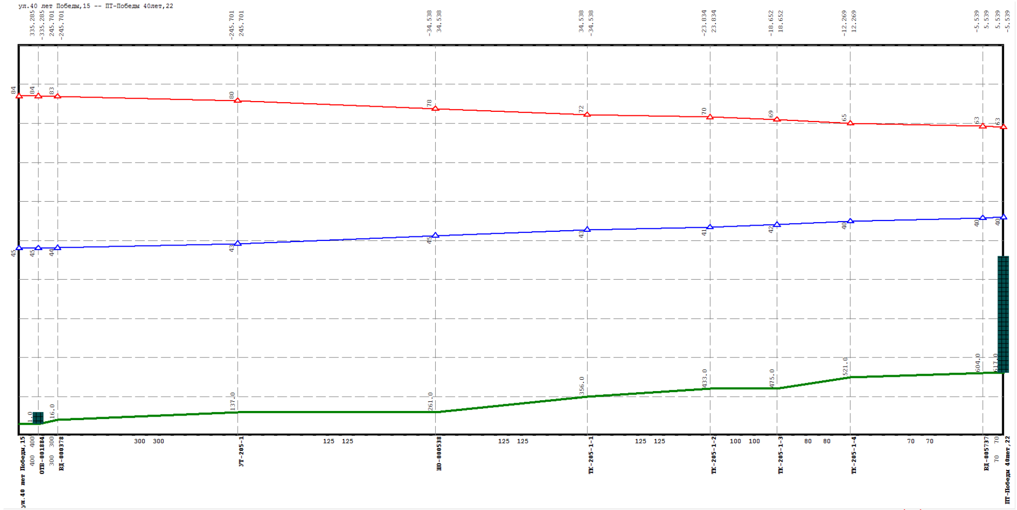
Рисунок Ошибка! Текст указанного стиля в документе отсутствует..46 Результат гидравлического расчета - график гидравлических режимов по пути теплоносителя от котельной 40 лет Победы, 15 до ПТ-Победа 40лет,22
