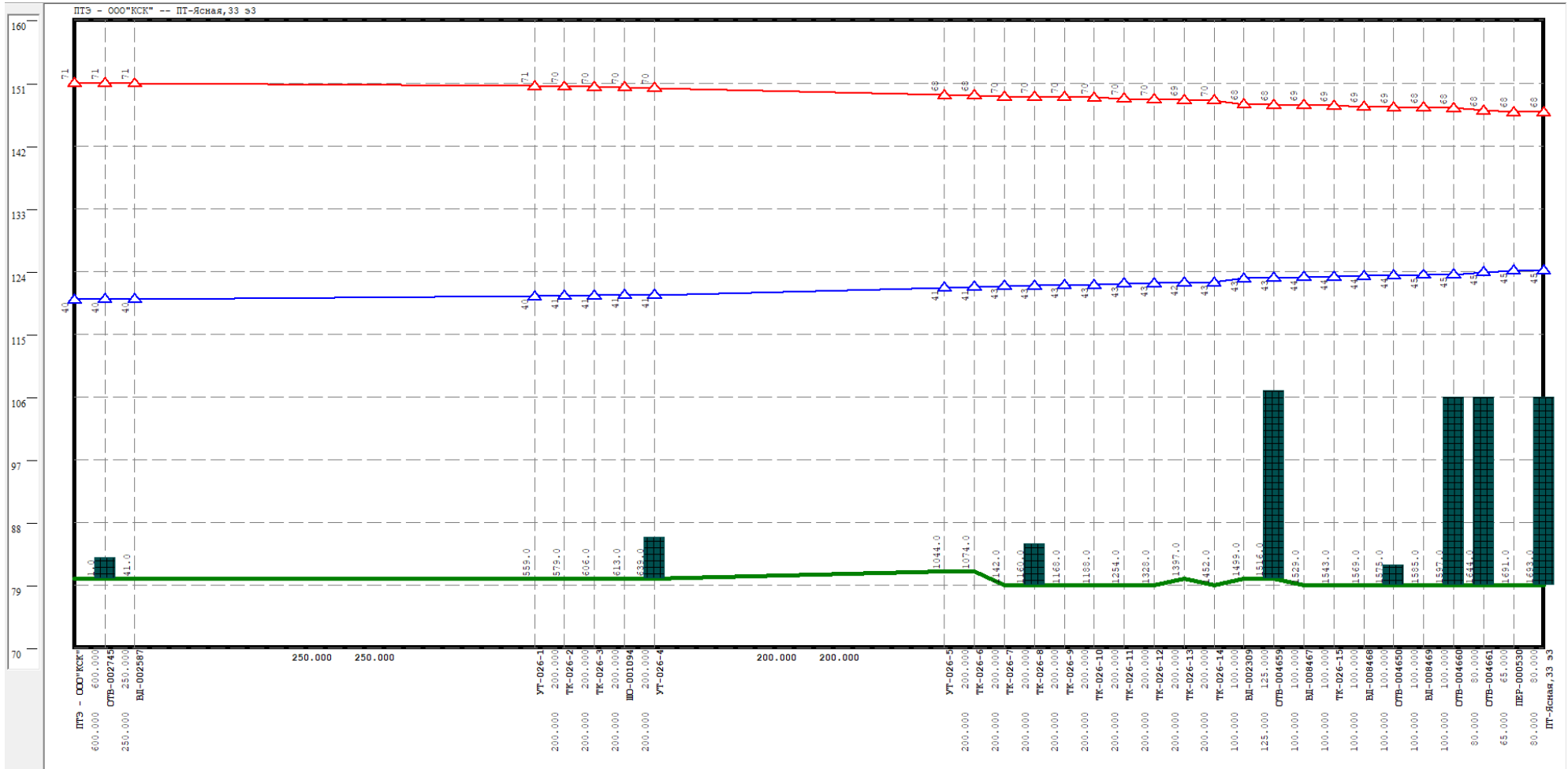
Рисунок Ошибка! Текст указанного стиля в документе отсутствует..60 Результат гидравлического расчета - график гидравлических режимов по пути теплоносителя от котельной Зайцева, 31 до ПТ-Ясная,33 э3
