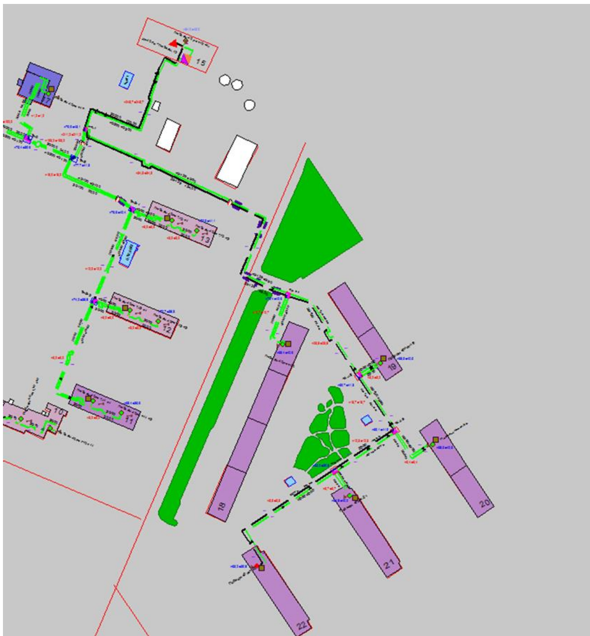
Рисунок Ошибка! Текст указанного стиля в документе отсутствует..45 Результат гидравлического расчета - расчетный путь теплоносителя от котельной 40 лет Победы, 15 до ПТ-Победы 40лет,22
