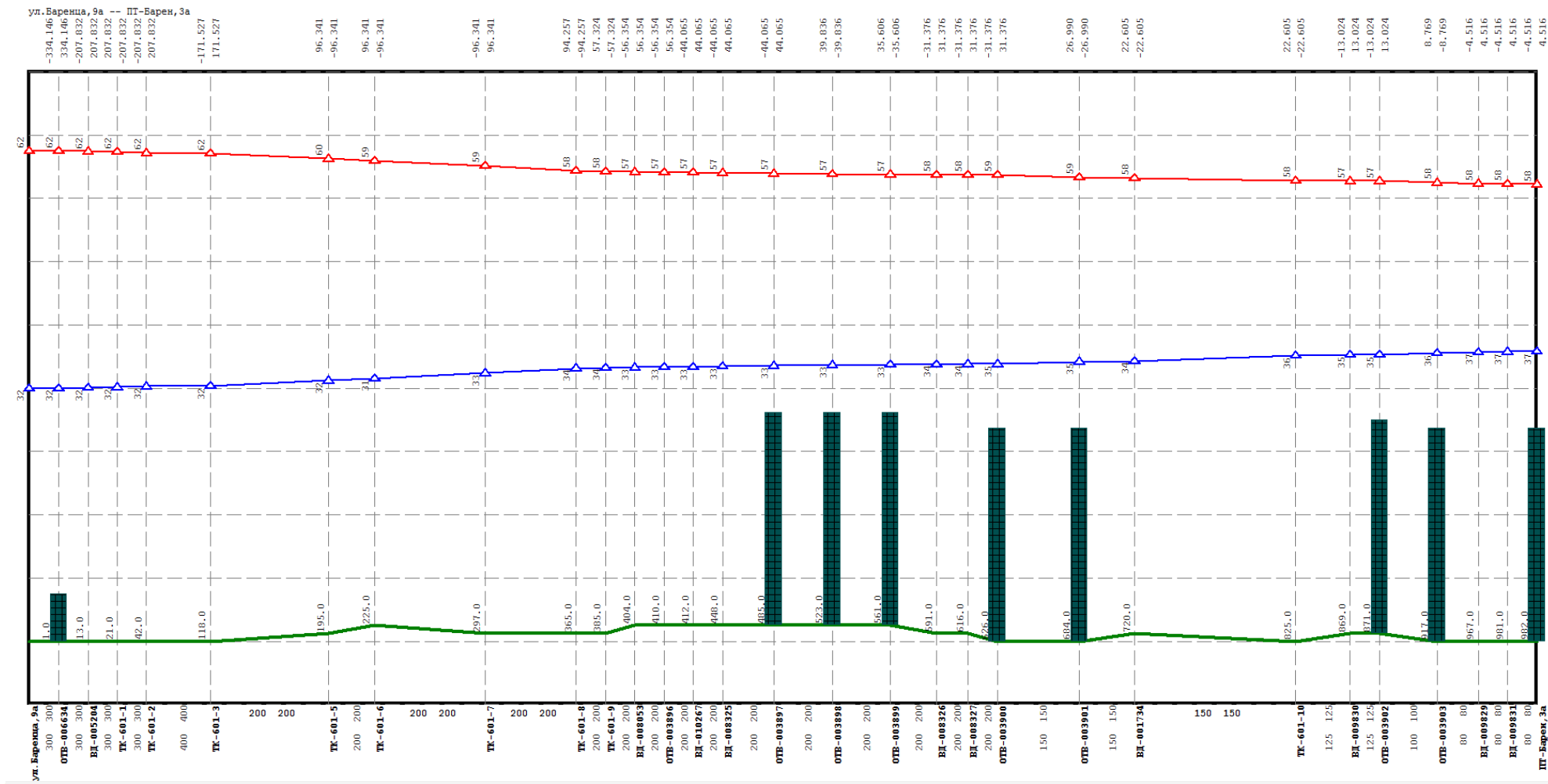
Рисунок Ошибка! Текст указанного стиля в документе отсутствует..70 Результат гидравлического расчета - график гидравлических режимов по пути теплоносителя от котельной Баренца, 9а до ПТ-Баренца, 3а
