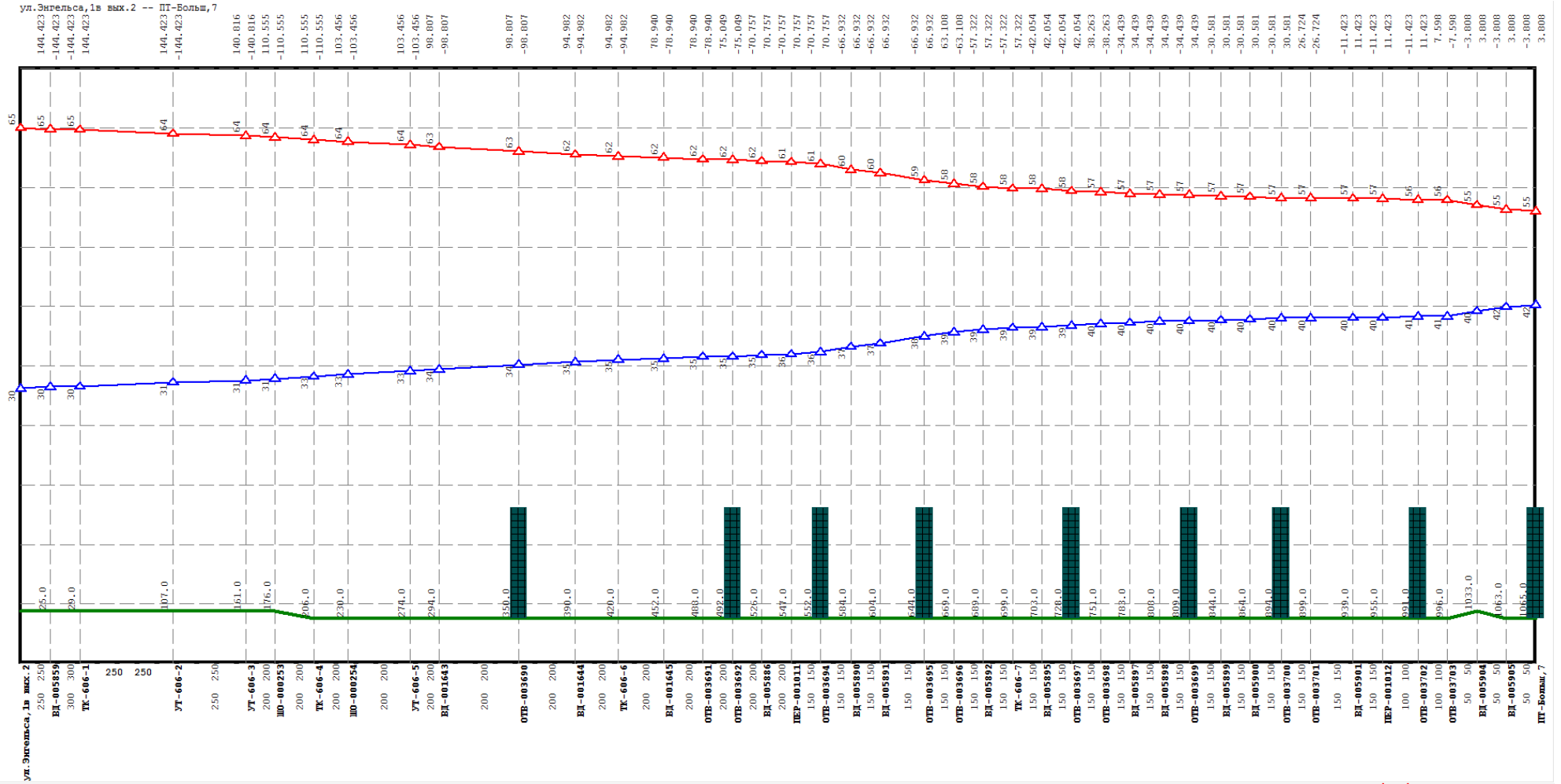
Рисунок Ошибка! Текст указанного стиля в документе отсутствует..6 Результат гидравлического расчета - график гидравлических режимов по пути теплоносителя от котельной Энгельса, 1-в до ПТ-Больш, 7
