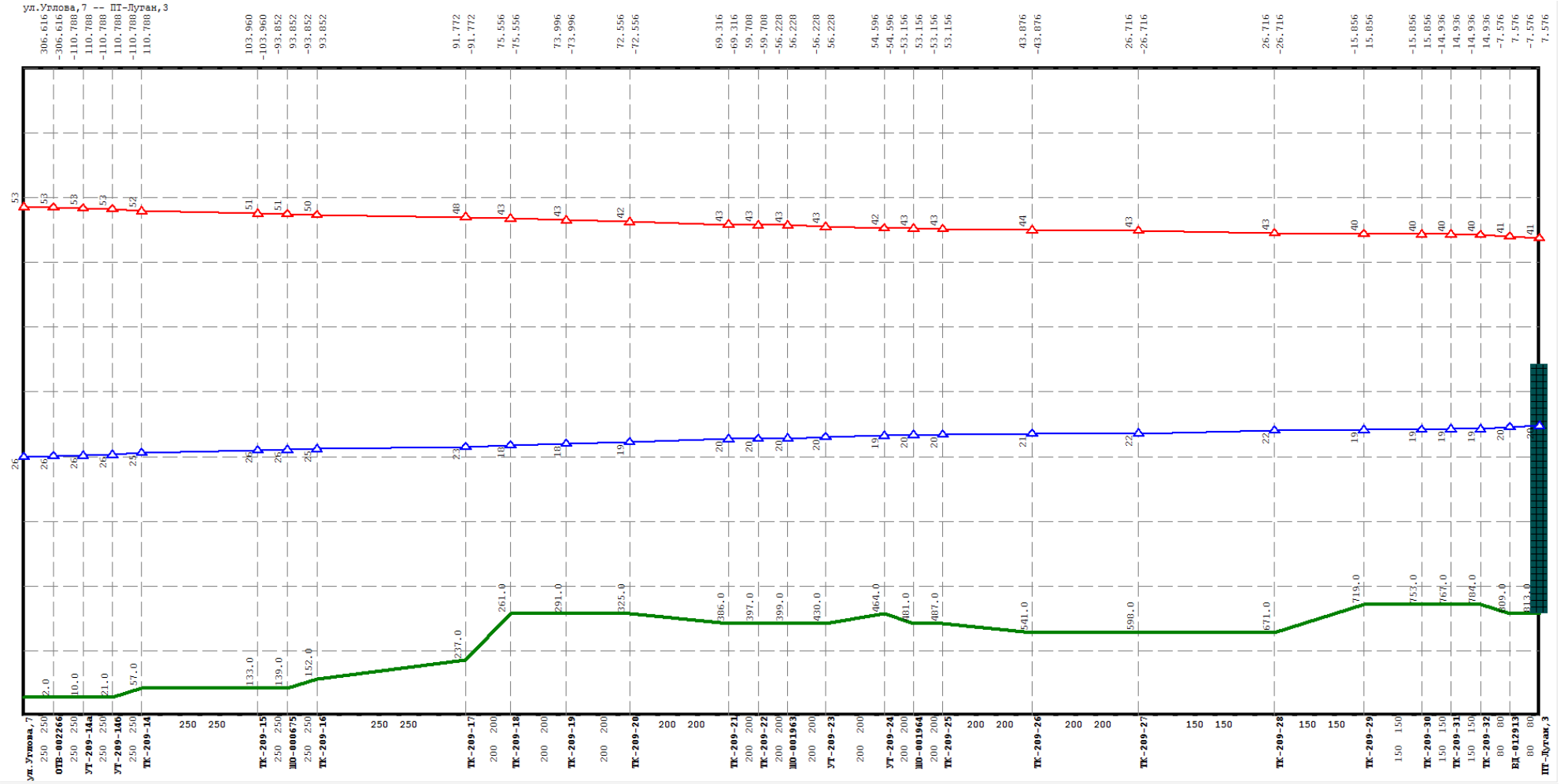
Рисунок Ошибка! Текст указанного стиля в документе отсутствует..108 Результат гидравлического расчета - график гидравлических режимов по пути теплоносителя от котельной ул. Углова, 7 до ПТ-Луган,3
