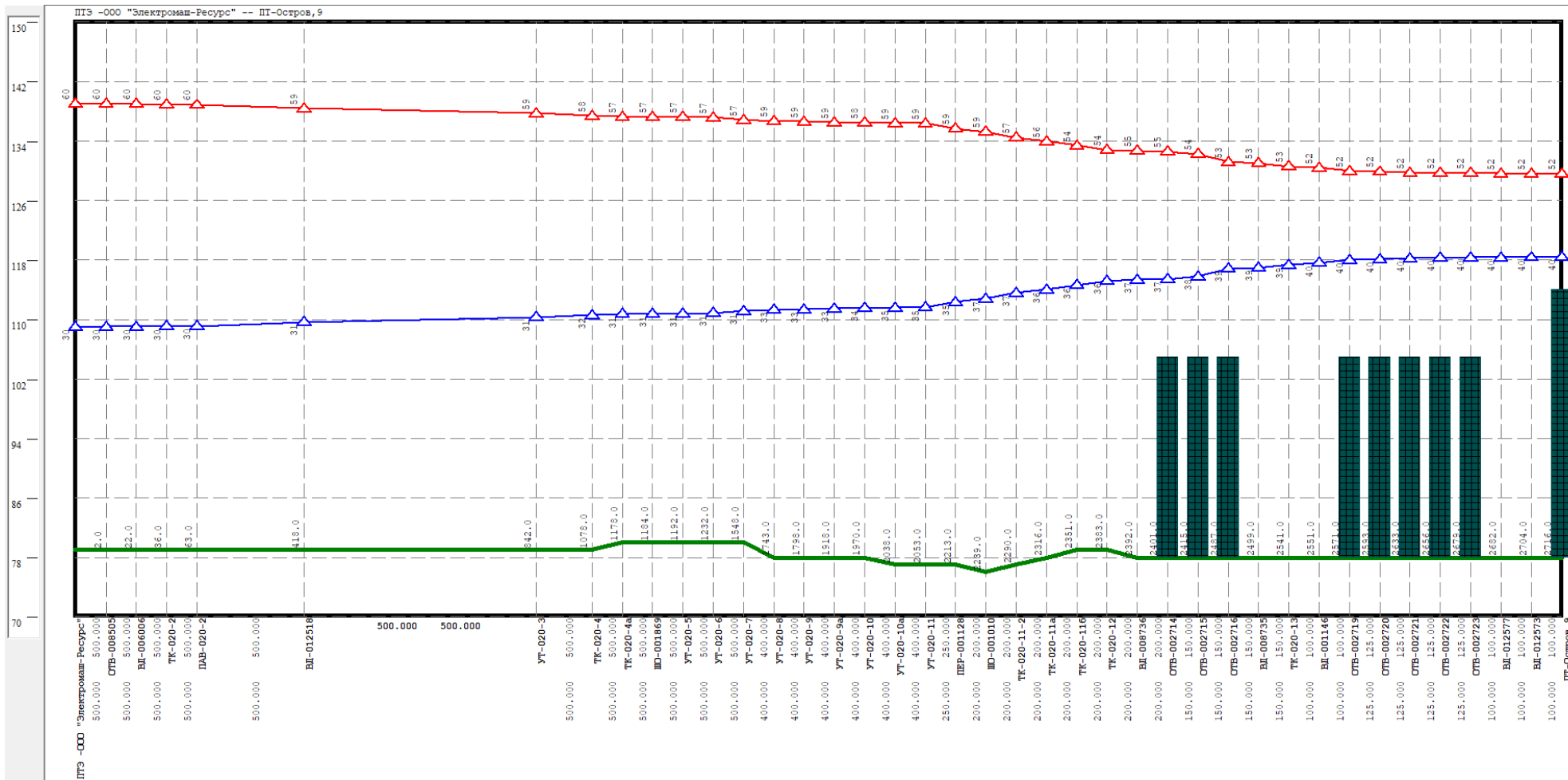
Рисунок Ошибка! Текст указанного стиля в документе отсутствует..96 Результат гидравлического расчета - график гидравлических режимов по пути теплоносителя от котельной Федосеенко, 64 до ПТ-Остров,9
