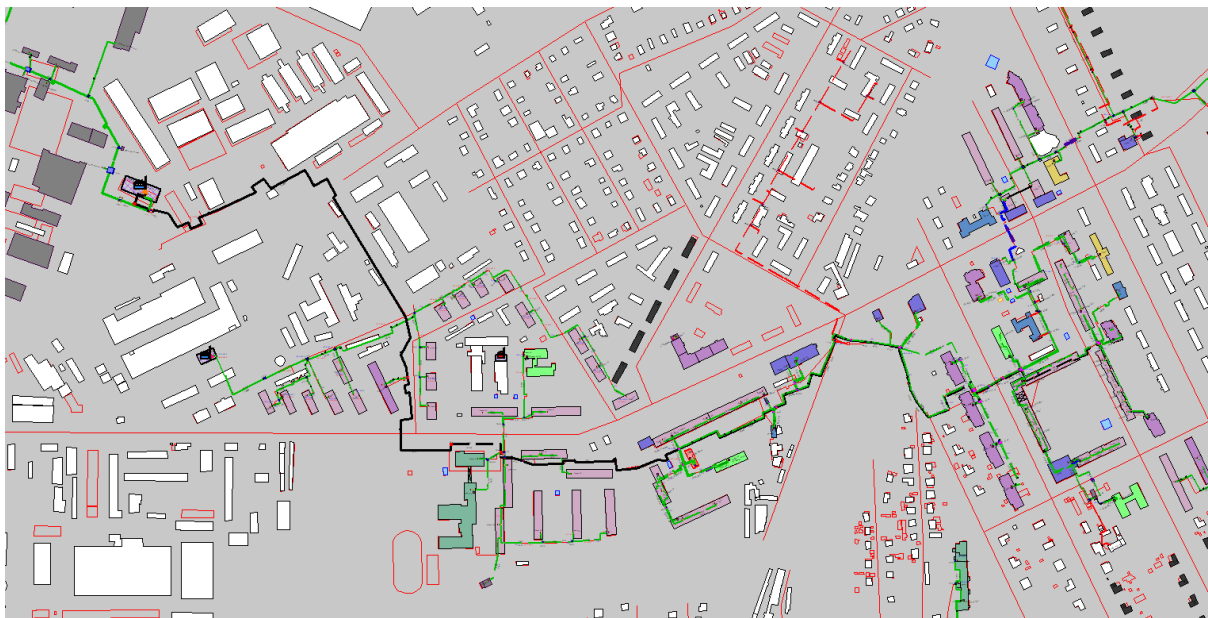
Рисунок Ошибка! Текст указанного стиля в документе отсутствует..95 Результат гидравлического расчета - расчетный путь теплоносителя от котельной Федосеенко, 64 до ПТ-Остров,9
