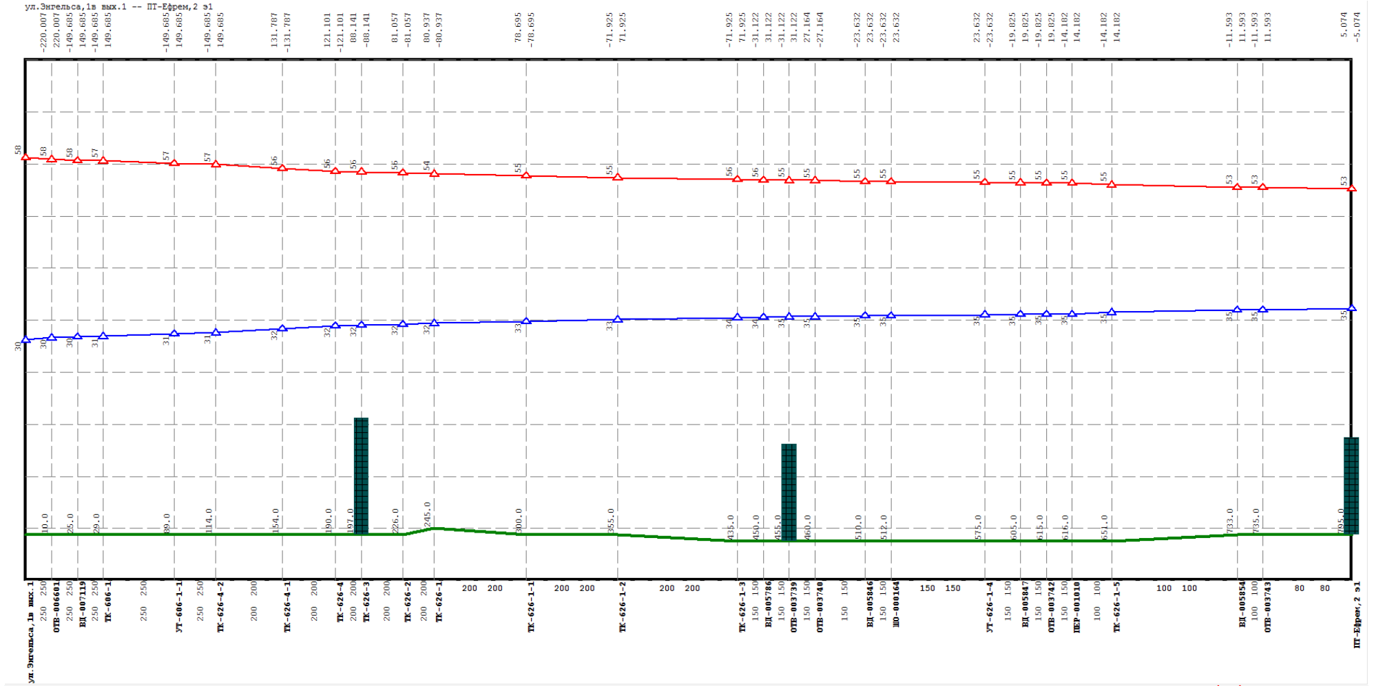
Рисунок 2. Результат гидравлического расчета - график гидравлических режимов по пути теплоносителя от котельной Энгельса, 1-в до ПТ-Ефрем, 2 э1
