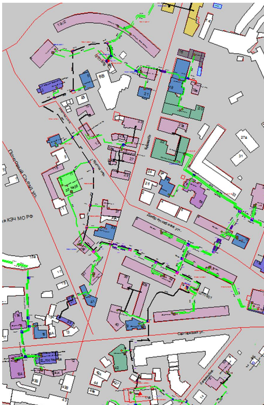
Рисунок Ошибка! Текст указанного стиля в документе отсутствует..25 Результат гидравлического расчета - расчетный путь теплоносителя от котельной Плотничный, 11 до ЦТП-602
