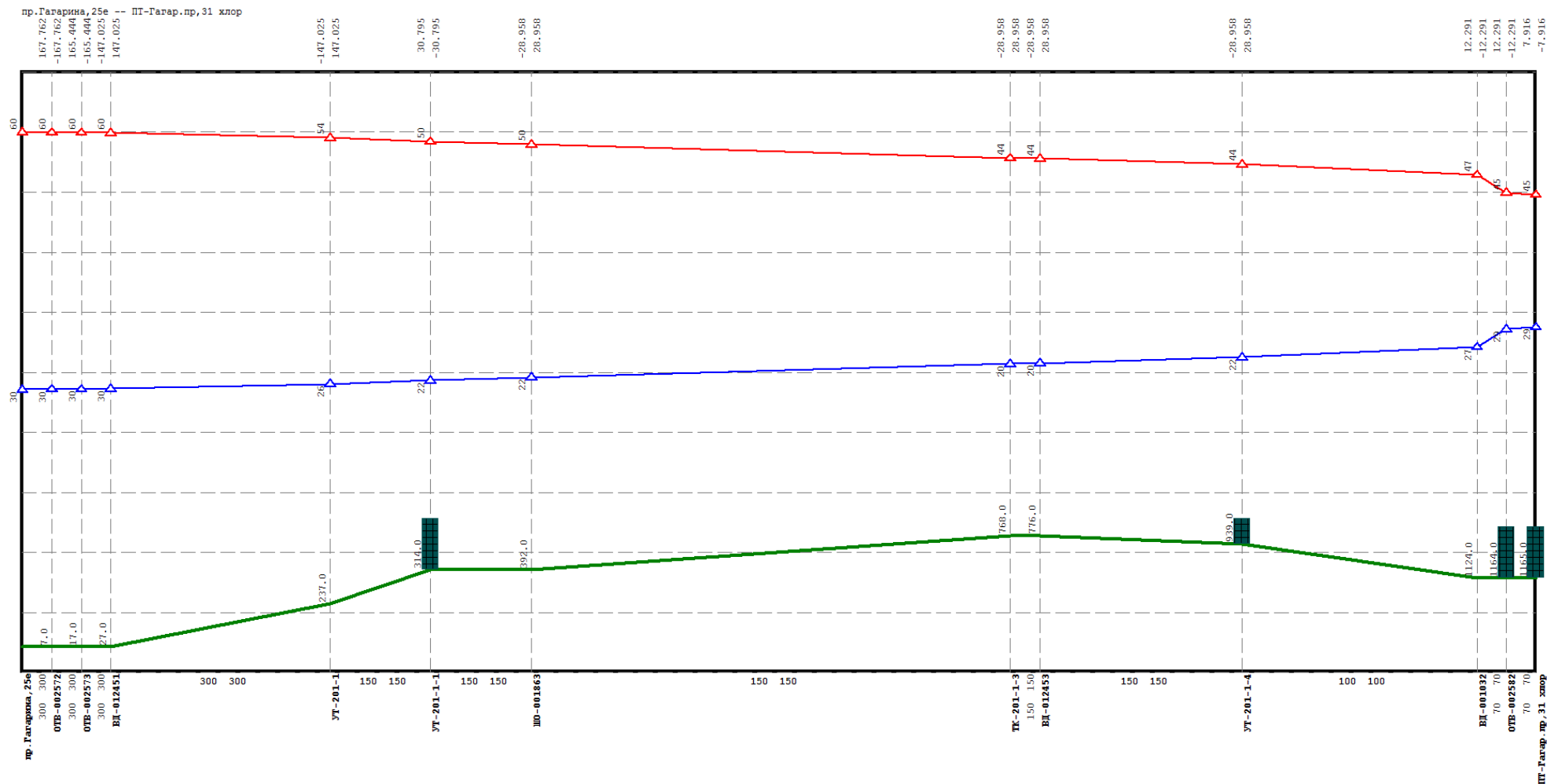
Рисунок Ошибка! Текст указанного стиля в документе отсутствует..54 Результат гидравлического расчета - график гидравлических режимов по пути теплоносителя от котельной Гагарина, 25-е до ПТ-Гагар. пр, 31 хлор
