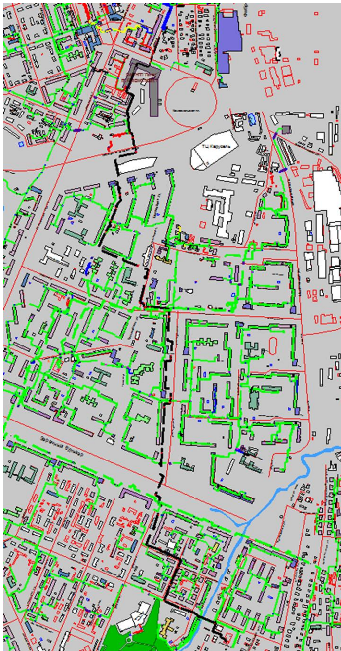
Рисунок Ошибка! Текст указанного стиля в документе отсутствует..65 Результат гидравлического расчета - расчетный путь теплоносителя от котельной Заводская, 19 до ПТ-Комсом.пл,3
