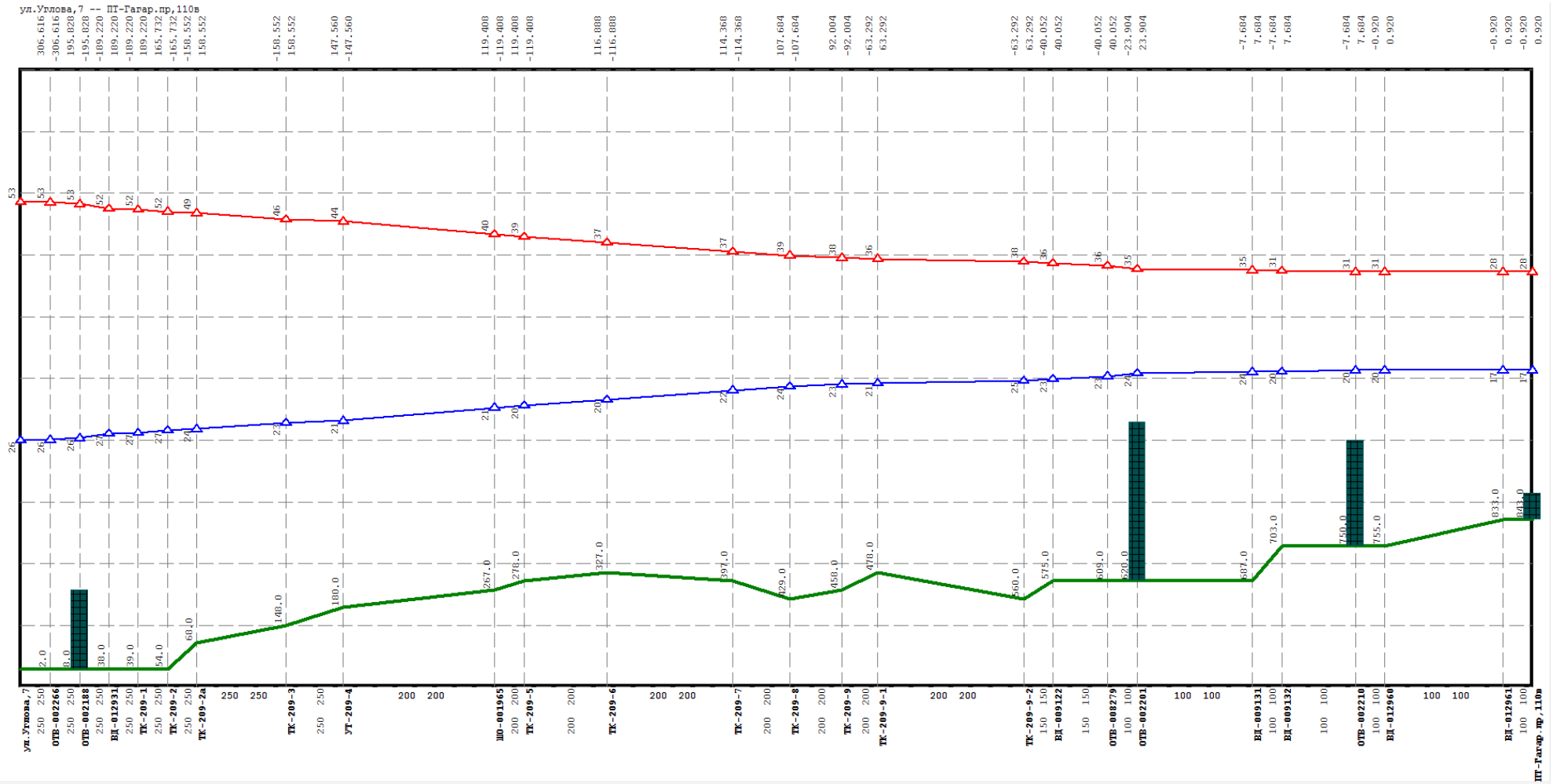
Рисунок Ошибка! Текст указанного стиля в документе отсутствует..106 Результат гидравлического расчета - график гидравлических режимов по пути теплоносителя от котельной Углова, 7 до ПТ-Гагар.пр,110в
