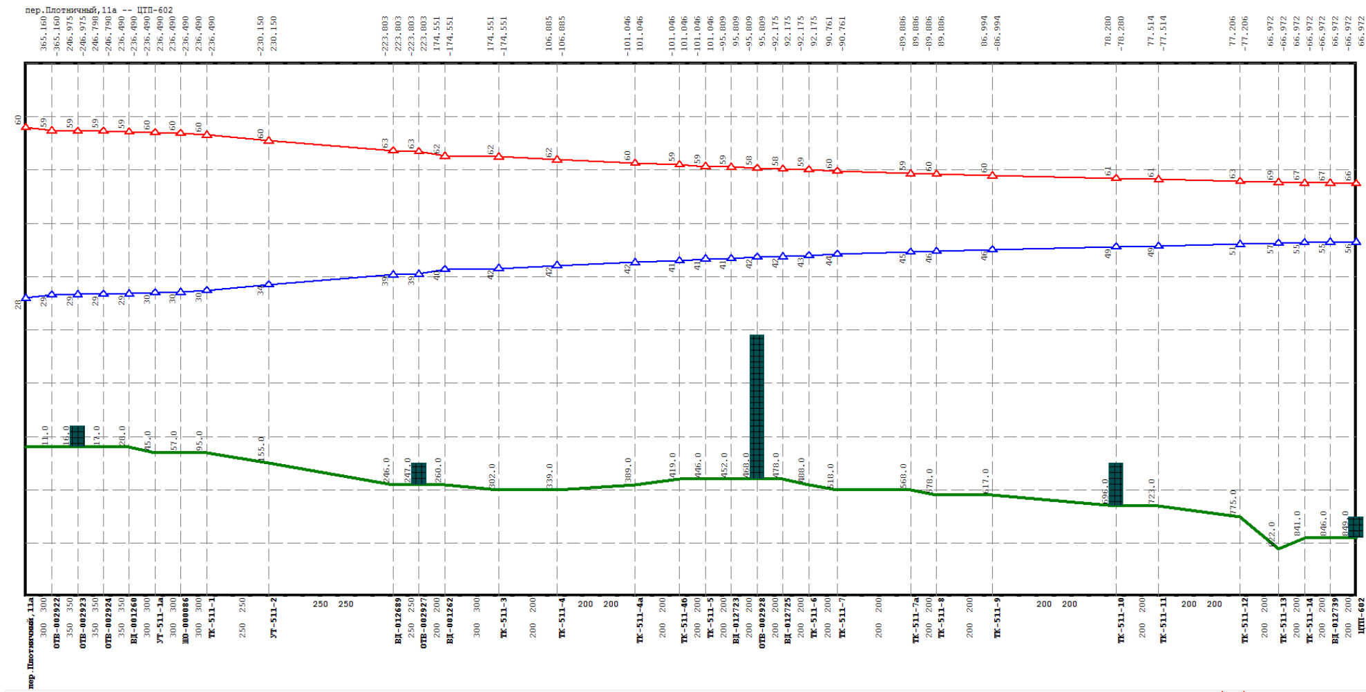
Рисунок Ошибка! Текст указанного стиля в документе отсутствует..26 Результат гидравлического расчета - график гидравлических режимов по пути теплоносителя от котельной Плотничиный, 11 до ЦТП-602
