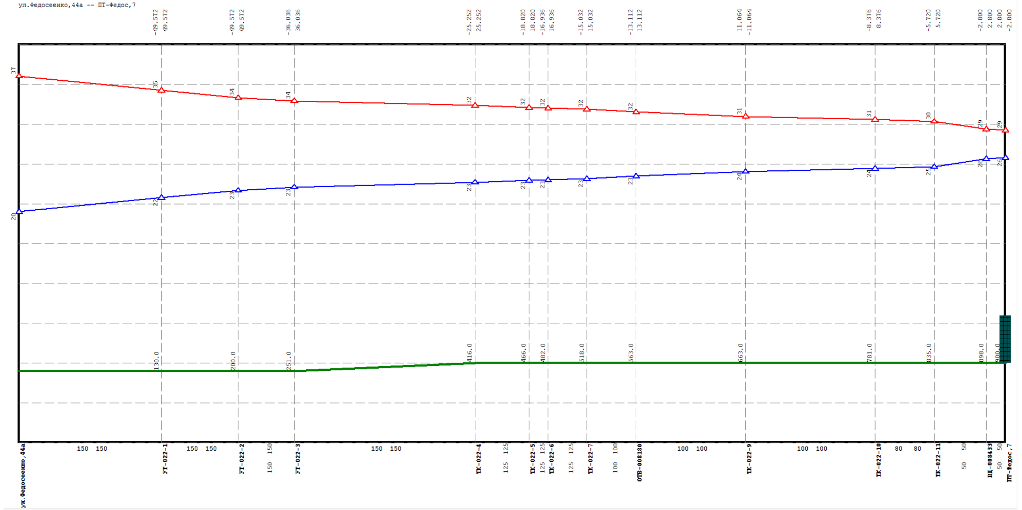
Рисунок Ошибка! Текст указанного стиля в документе отсутствует..92 Результат гидравлического расчета - график гидравлических режимов по пути теплоносителя от котельной Федосеевко, 44а до ПТ-Федос,7
