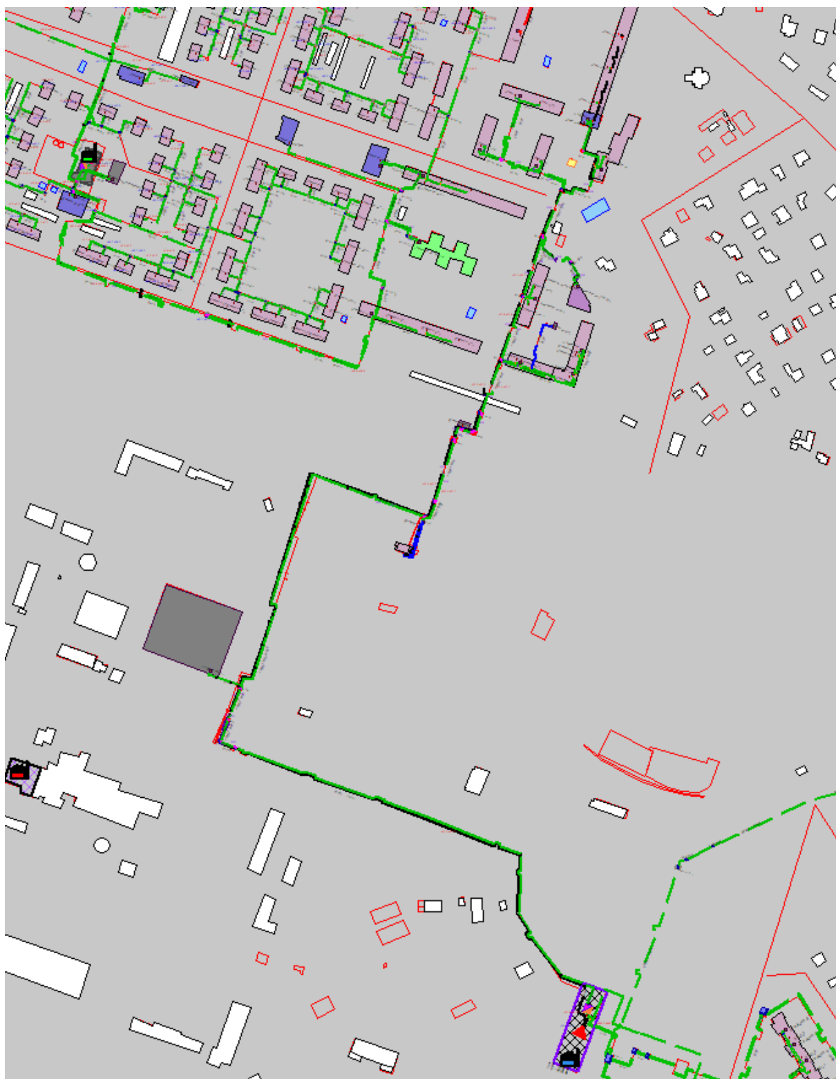
Рисунок Ошибка! Текст указанного стиля в документе отсутствует..59 Результат гидравлического расчета - расчетный путь теплоносителя от котельной Зайцева, 31 до ПТ-Ясная,33 э3
